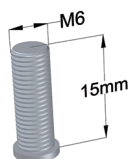
EARTH STUD
