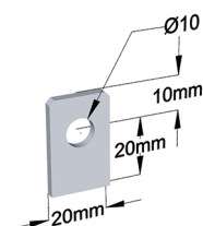
EARTH LUG
